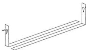
BARS Barres courtes ajustables (2) de 13 1/2" à 21 3/4" 343 mm à 553 mm
